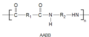
Poliamidas
